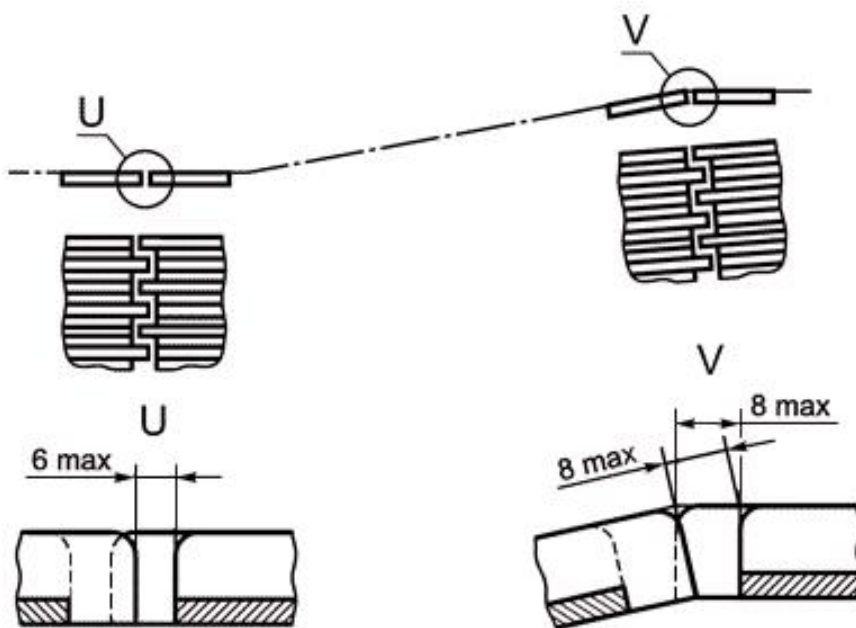
Рисунок 7 - Пластины, зазор и глубина входа выступов в углубления смежной пластины (пластинчатый пассажирский конвейер с выступами и впадинами на передних и задних краях пластин) у нижней и верхней входных площадок и в месте перехода от горизонтального участка к наклонному
